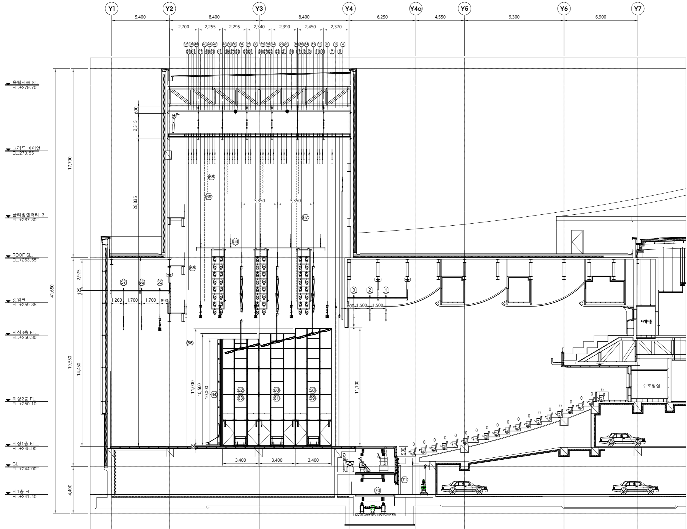
무대기계장치 단면도
